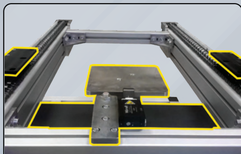
Positionneur pneumatique
